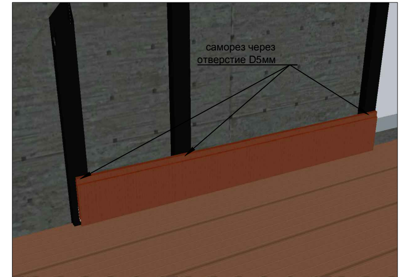
монтаж первой доски
