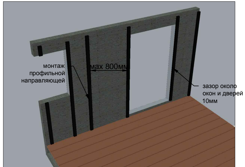
подготовка основания для укладки сайдинга
