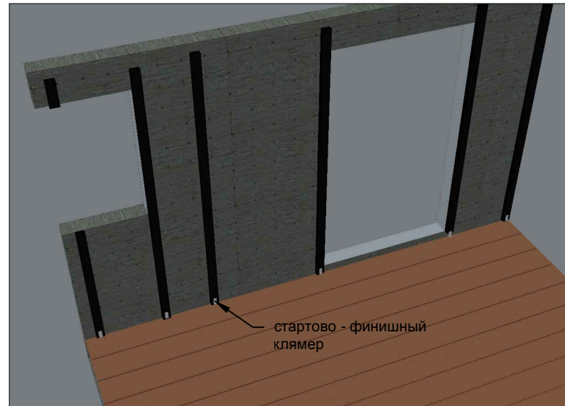
монтаж стартово-финишных клямеров для фиксации первой доски
