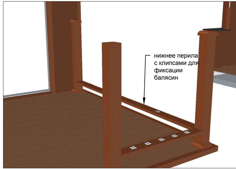
сборка перил №2
