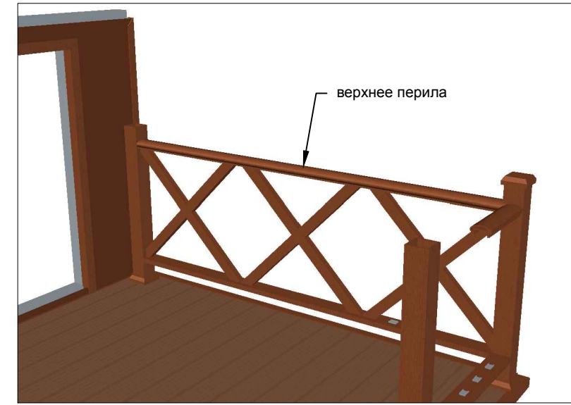
сборка перил №2
