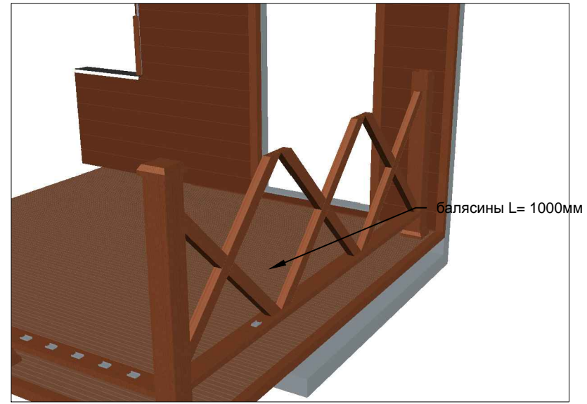
сборка перил №2
