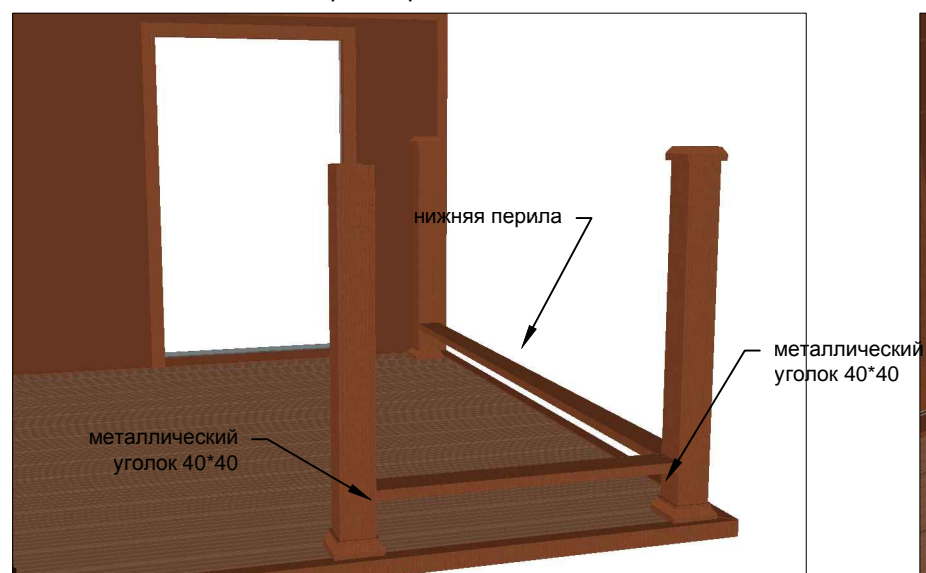
сборка перил
