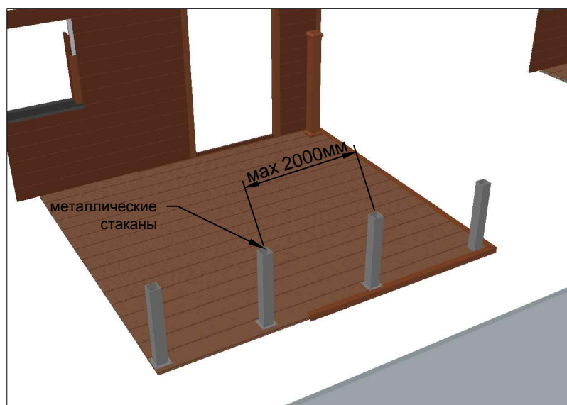
монтаж алюминиевых колонн
