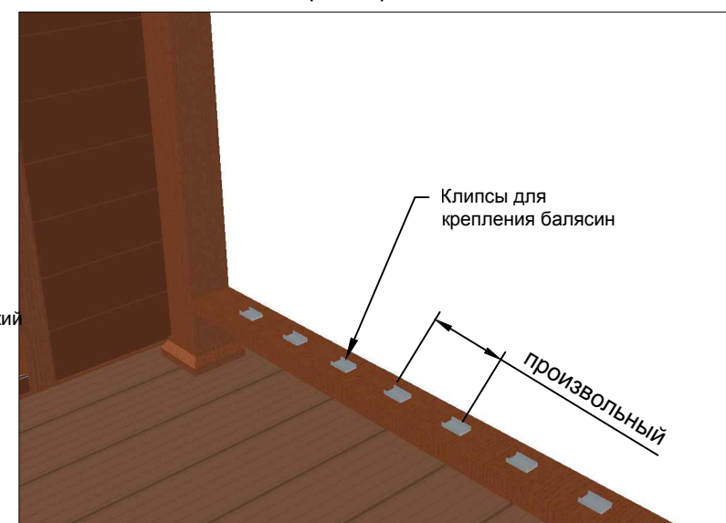
сборка перил
