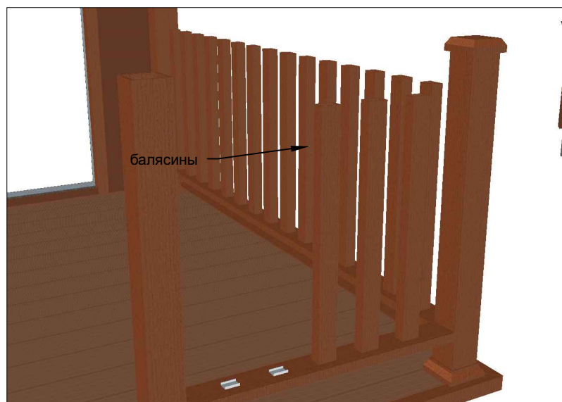
сборка перил
